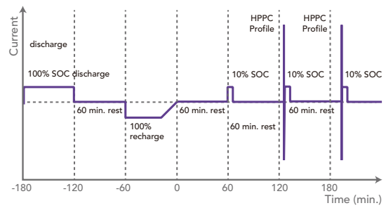
HPPC Test
